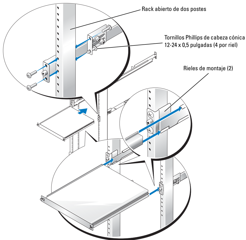
Figura 5-14. Instalación de los rieles de montaje para una configuración de montaje a ras
