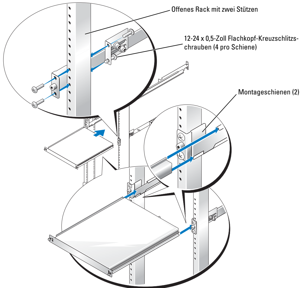
Abbildung 3-14. Einbau der Montageschienen mit bündiger Montage
